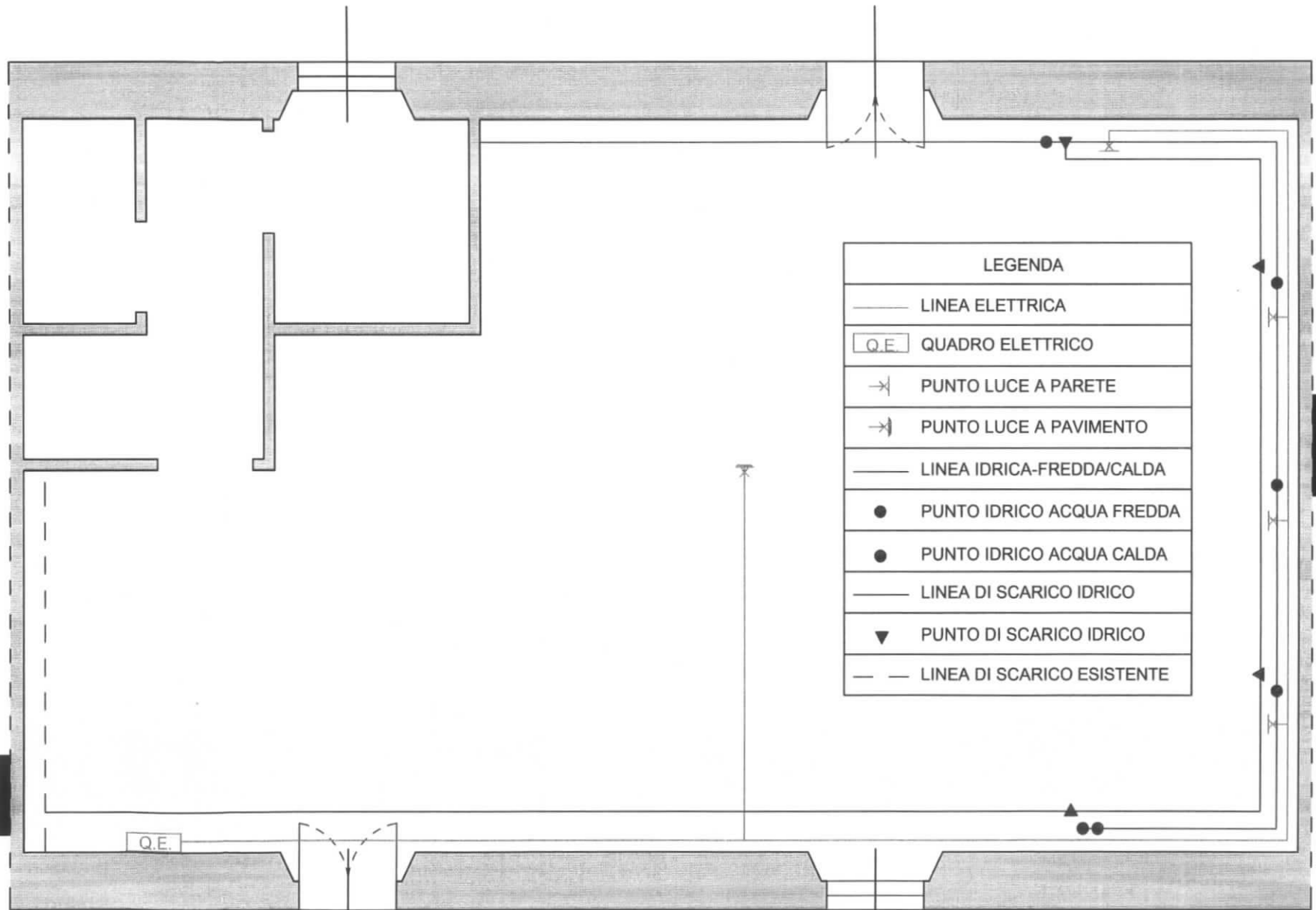
PIANTA LABORATORIO RAPP. 1/50
