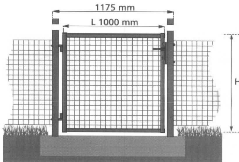
Tipologia cancelletto
